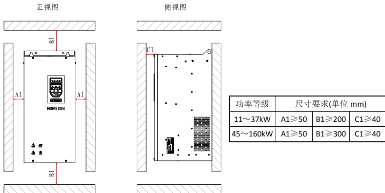
图3-2 单台机器 (Hope130G11T4~Hope130G160T4) 安装间隔
